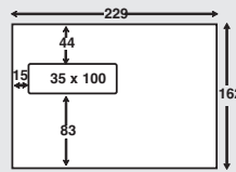
Vindu nr. 16. C5 høyt vindu venstre
