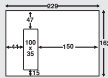
Vindu nr. 14. C5 tverrstilt vindu
