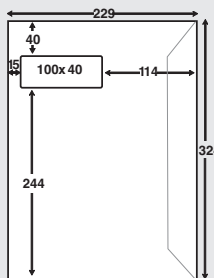
V2-Tverrstilt vindu C4
