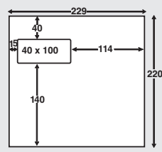
Vindu nr. 21. 220 x 229 høyt vindu venstre
