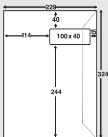
H2-Tverrstilt vindu C4
