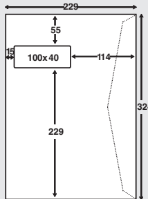
Vindu nr. 17. C4
